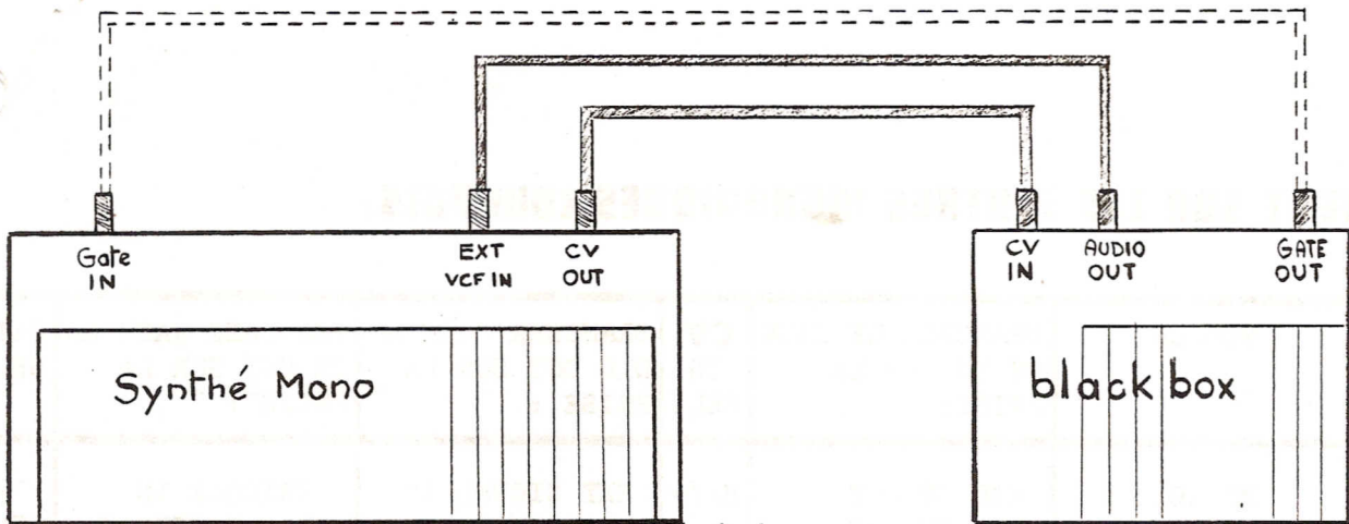
CONNECTION SUR UN SYNTHETISEUR
