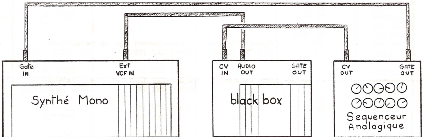
CONNECTION SUR UN SYNTHÉ + SEQ. ANALOGIQUE
