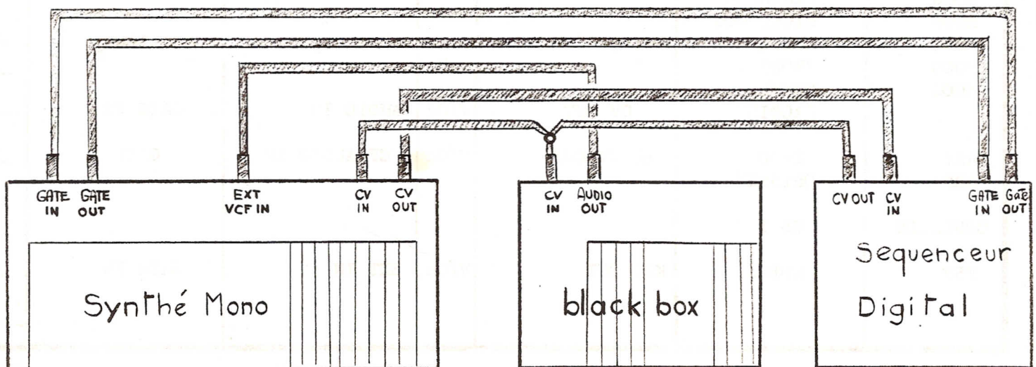
CONNECTION SUR UN SYNTHÉ + SEQUENCEUR DIGITAL
