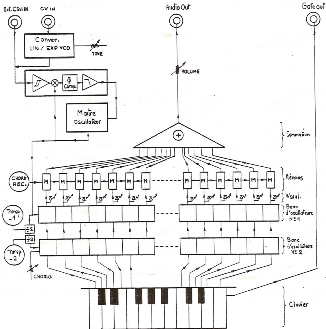
SCHEMA SYNOPTIQUE
